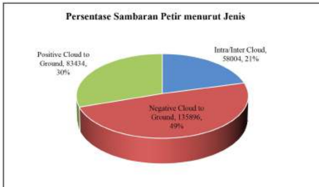
Gambar 5. Total Sambaran Menurut Jenis Muatan
