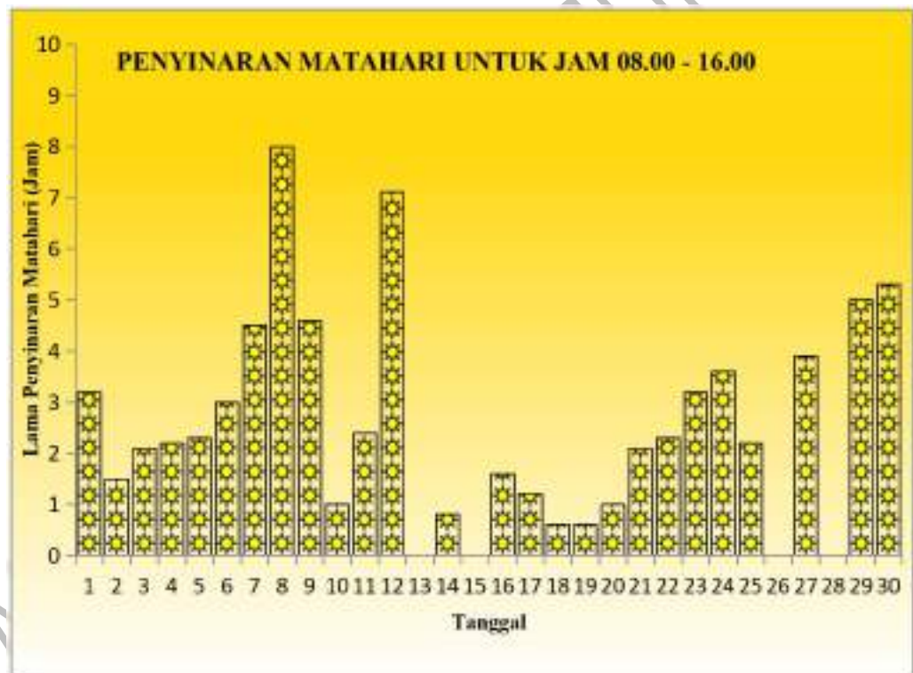
Gambar 17. Grafik Lama Penyinaran Matahari
