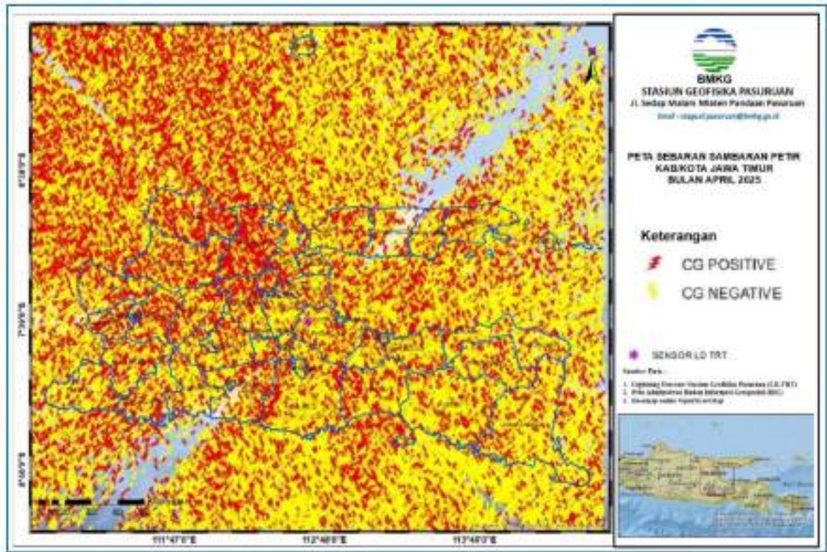
Gambar 9. Peta Intensitas Sambaran Petir di Wilayah Kabupaten Pasuruan dan Sekitarnya Bulan April 2025.
