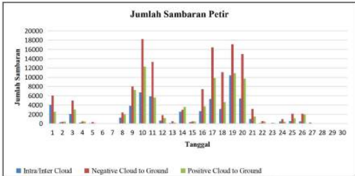
Gambar 6. Jumlah Sambaran Petir
