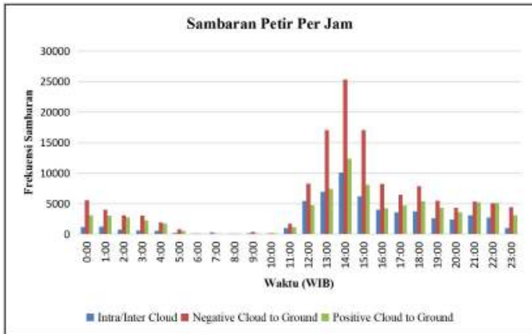
Gambar 8. Jumlah Sambaran Petir Per Jam
