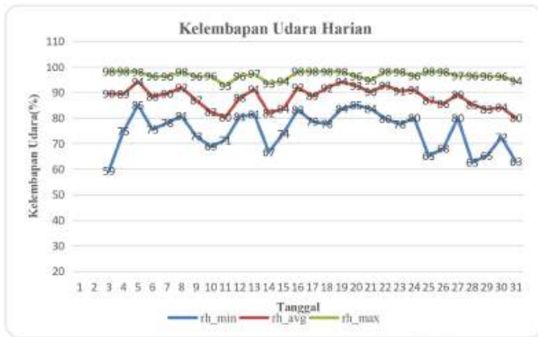
Gambar 15. Grafik Kelembapan Udara Harian
