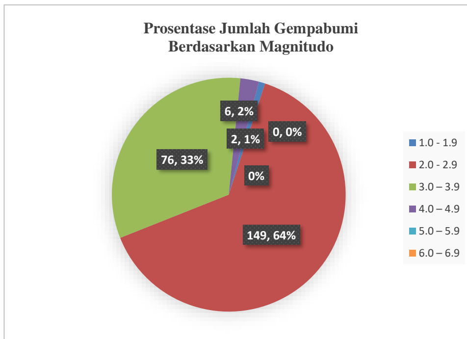
Gambar 2. Frekuensi Gempabumi Berdasarkan Magnitudo
