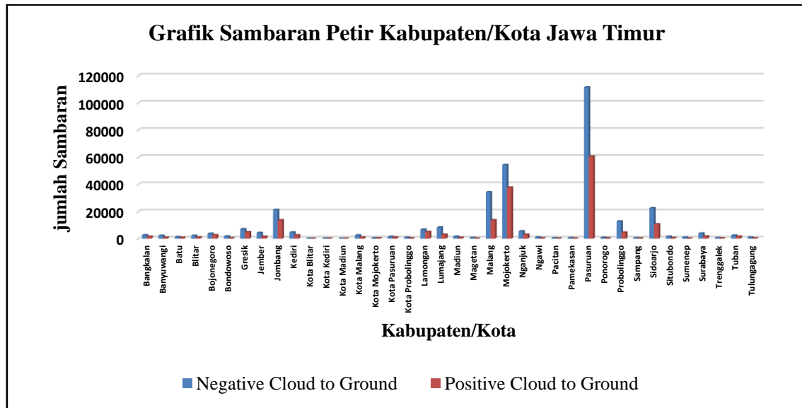
Gambar 7. Grafik Jumlah Sambaran Petir Wilayah Jawa Timur
