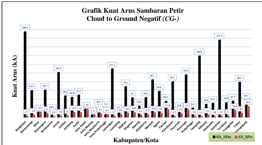
Gambar 15. Grafik Kuat Arus Sambaran Petir Cloud to Ground Negatif (CG-)
