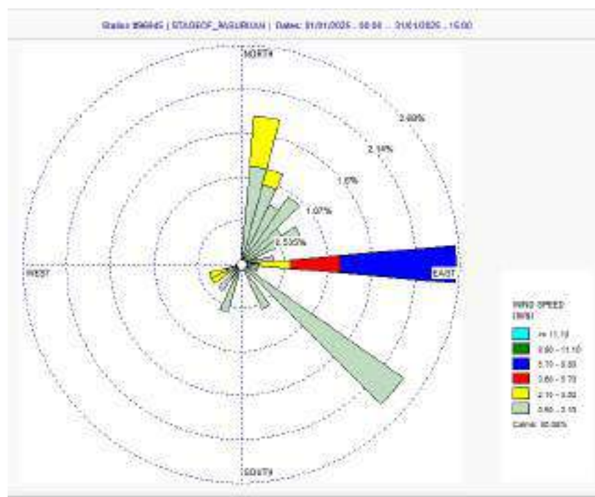
Gambar 18. Grafik Wind Rose
