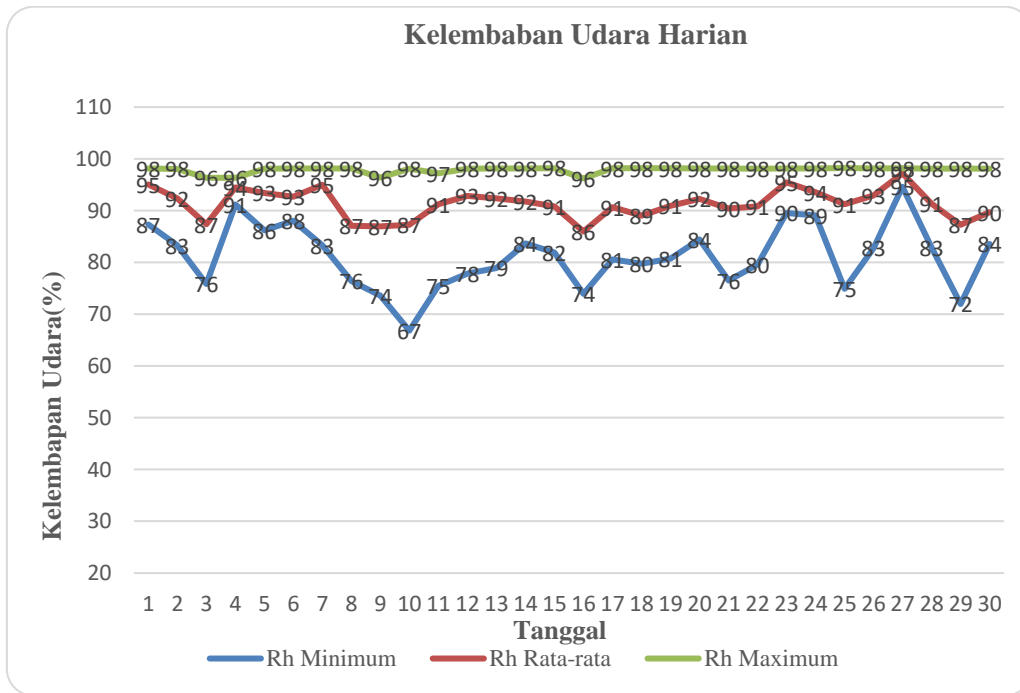
Gambar 17. Grafik Kelembapan Udara Harian
