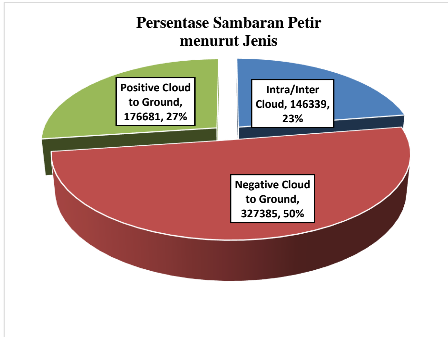
Gambar 5. Total Sambaran Menurut Jenis Muatan
