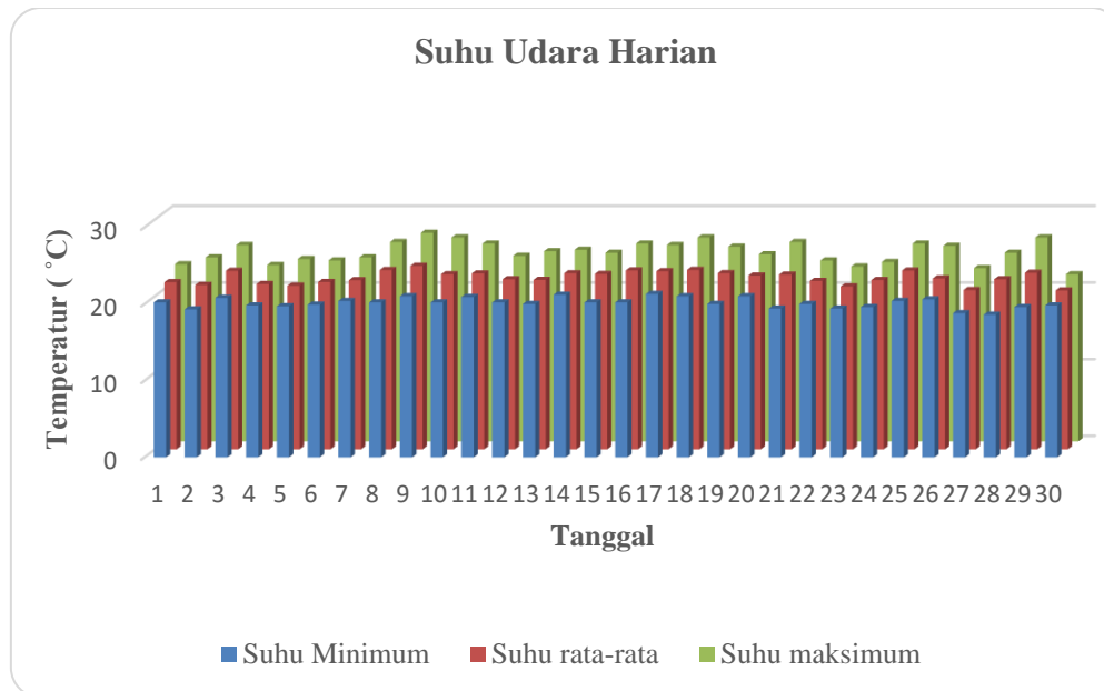
Gambar 16. Grafik Suhu Udara Harian
