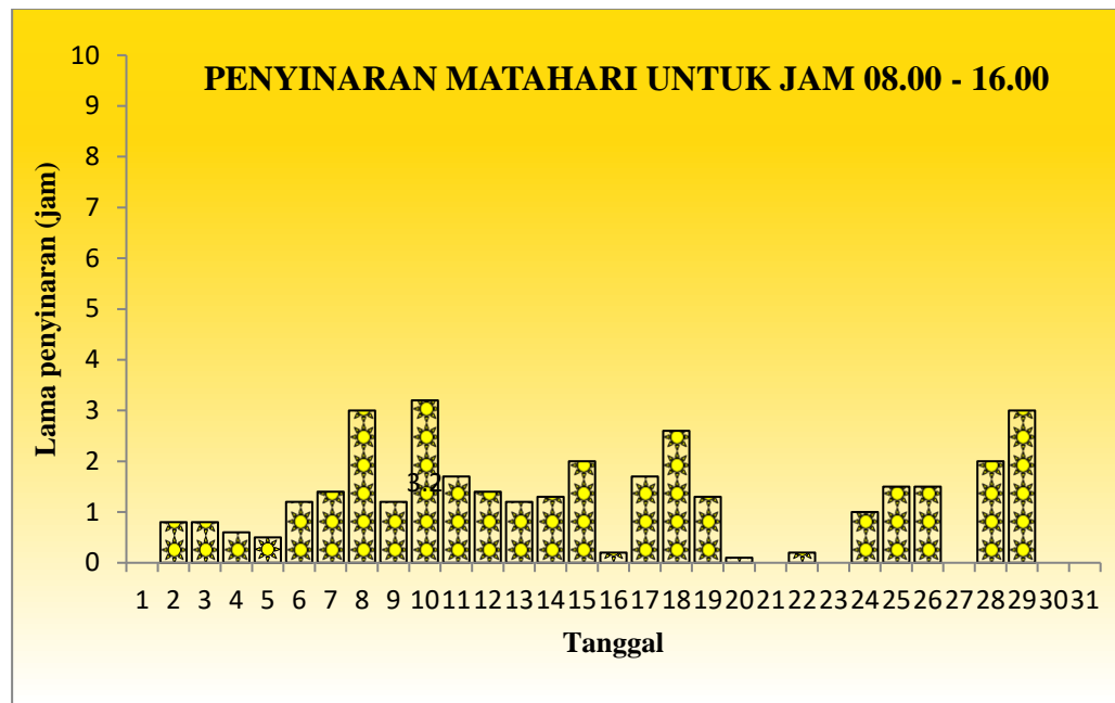
Gambar 19. Grafik Lama Penyinaran Matahari
