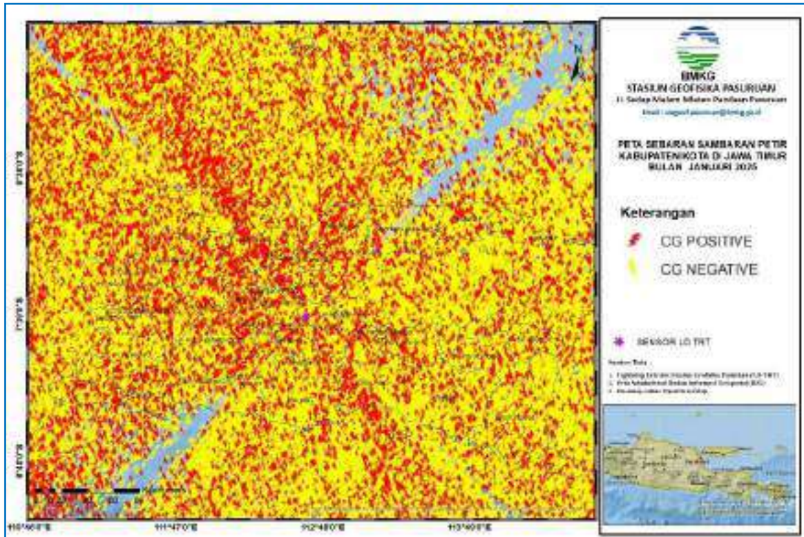
Gambar 9. Peta Intensitas Sambaran Petir di Wilayah Kabupaten Pasuruan dan Sekitarnya Bulan Januari 2025.
